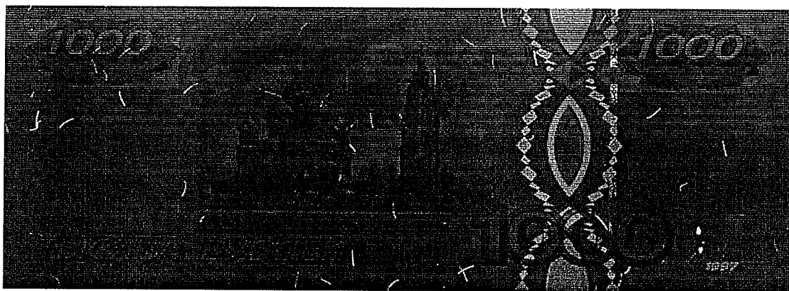
Рис. 10 Люминесценция
